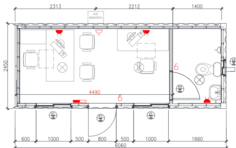
PLANTA REFERENCIAL COB 20'
