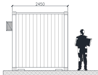
ELEVACIÓN LATERAL
