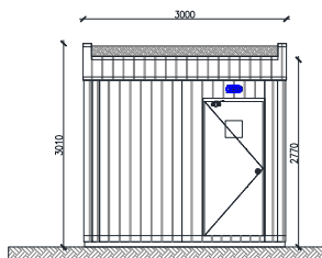
ELEVACIÓN VISTA - A ESC: 1/50
