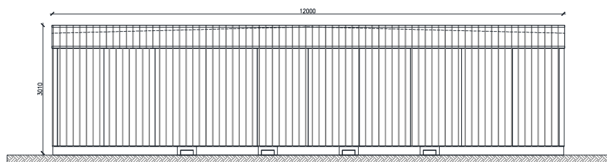
ELEVACIÓN VISTA - B ESC: 1/50
