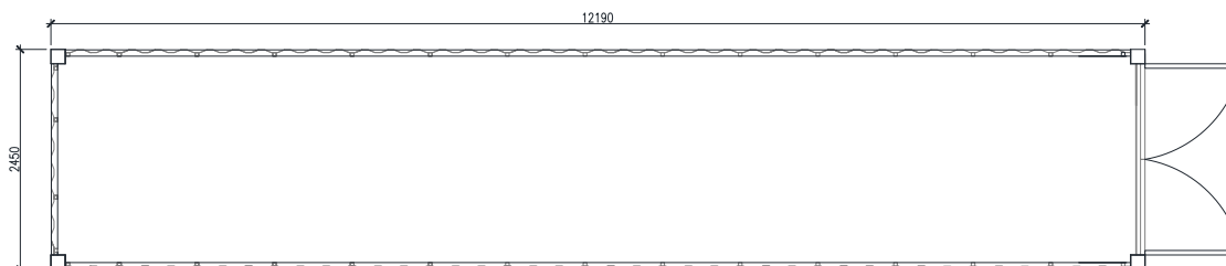
PLANTA CONTENEDOR DRY 40'
