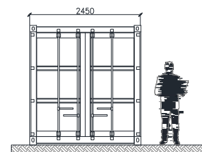
ELEVACIÓN LATERAL ESD: 1/50
