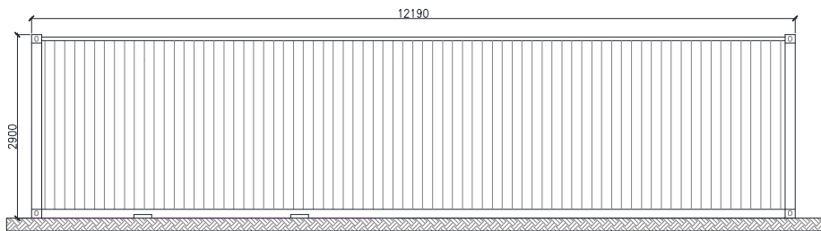
ELEVACIÓN FRONTAL
