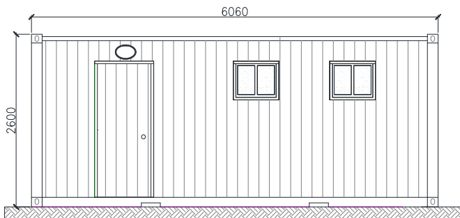
ELEVACIÓN FRONTAL
