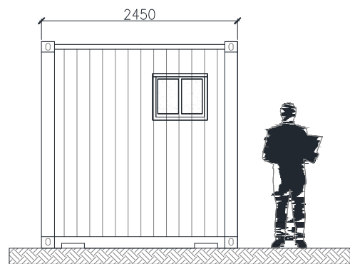
ELEVACIÓN LATERAL
