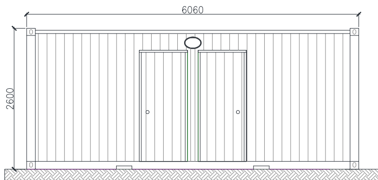
ELEVACIÓN FRONTAL
